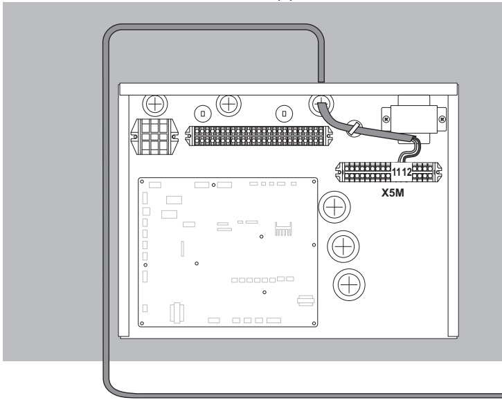
EHVH/X*(U)*E* + EHVZ*E*
